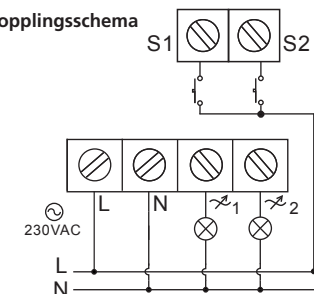
Kopplingschema
